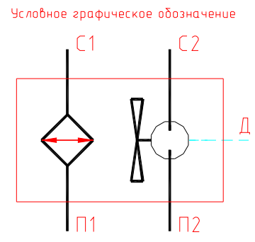
Рис. 39 Установка маслоохладительная Fig. 39 Oil Cooler Installation
