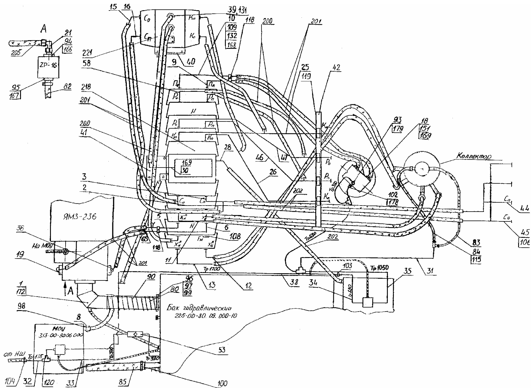
Рис. 18 Трубопроводы на поворотной платформе Fig. 18 Pippings on Slewing Turntable
