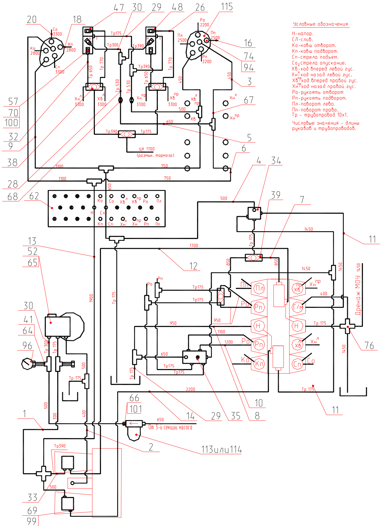
Рис. 36.1 Гидроуправление на поворотной платформе (монтажная схема) (с гидравликой ПСМ) Fig. 36.1 Hydraulic control on slewing turntable (assembly diagram) (PCM hydraulics)
