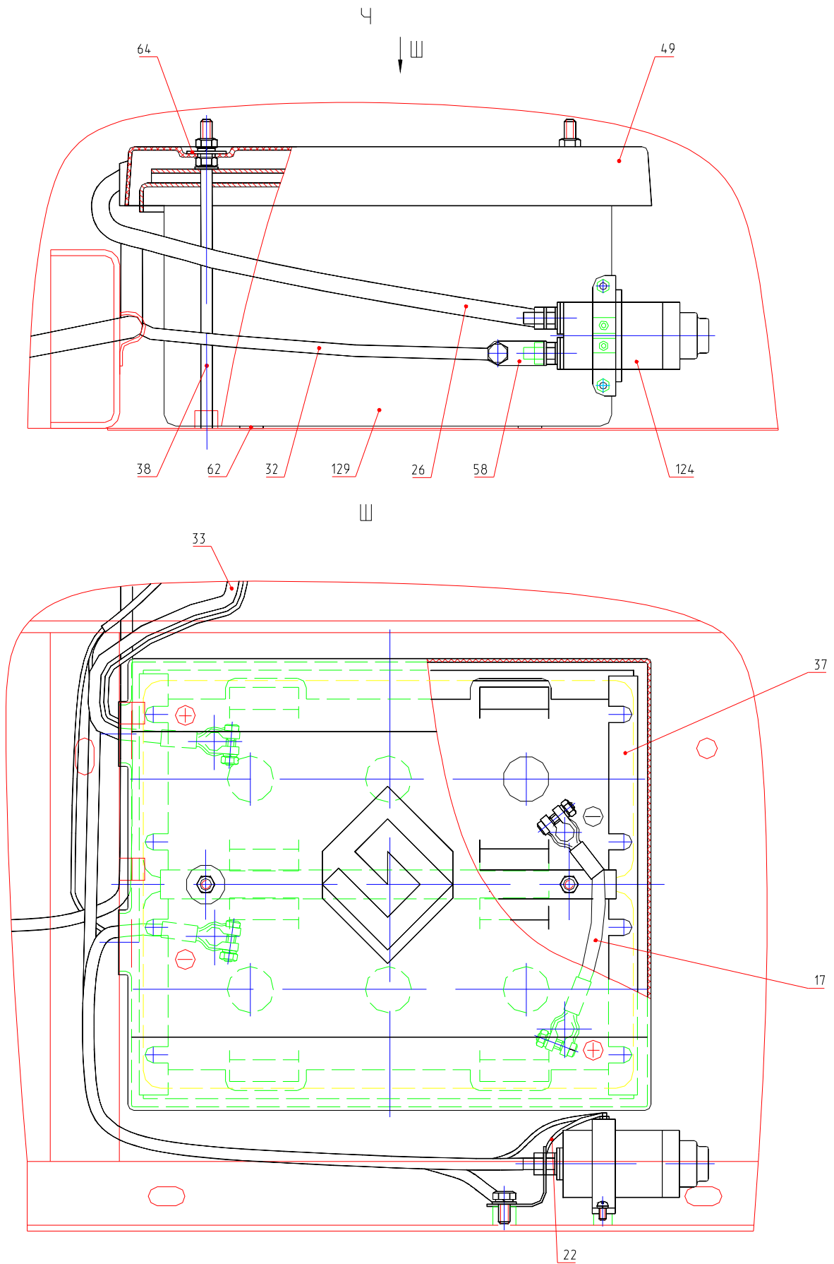
Рис. 63.6 Электрооборудование Fig. 63.6 Electric Equipment
