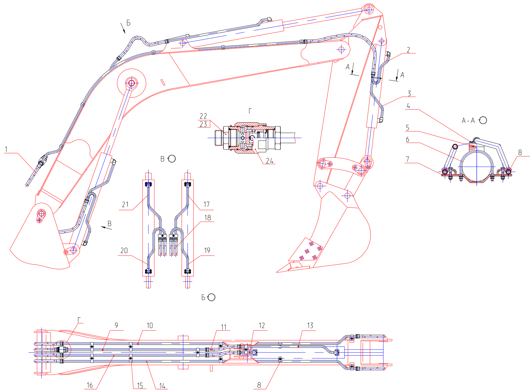
Рис. 48 Трубопроводы рабочего оборудования Fig. 48 Backhoe Equipment Pipings
