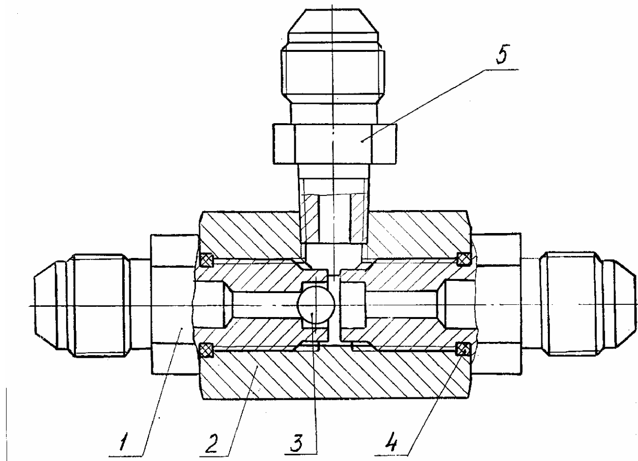
Рис. 39 Клапан «ИЛИ» Fig. 39 Valve «OR»
