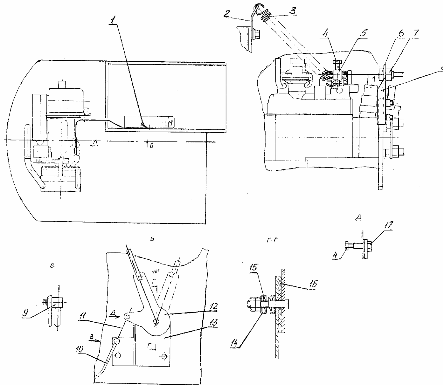
Рис. 10 Управление двигателем Fig. 10 Diesel control
