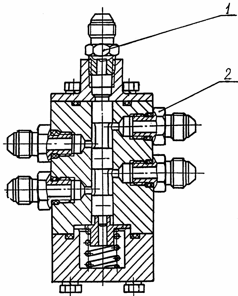
Рис. 37 Гидрораспределитель Fig. 37 Hydraulic Distributor
