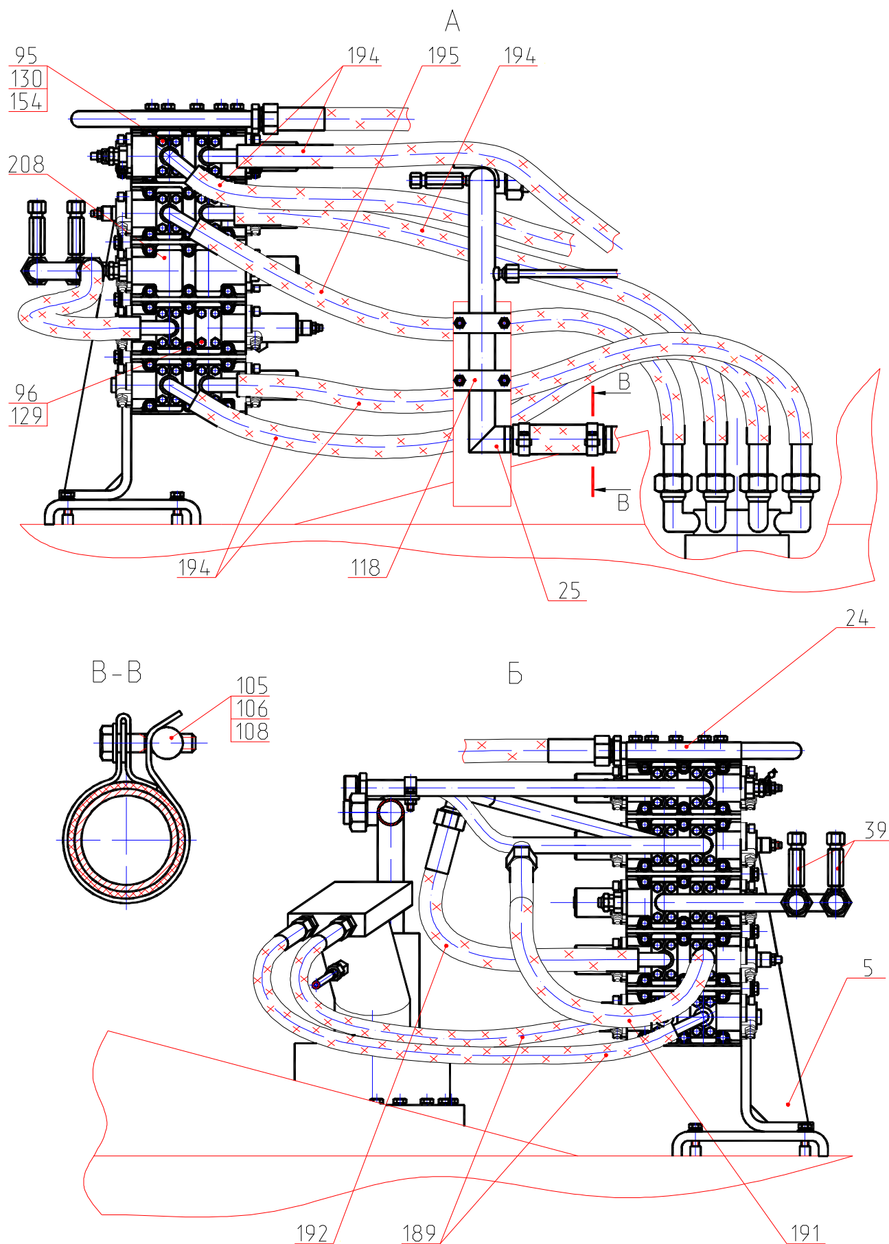
Рис. 27.2 Трубопроводы на поворотной платформе Fig. 27.2 Piping on Slewing Turntable
