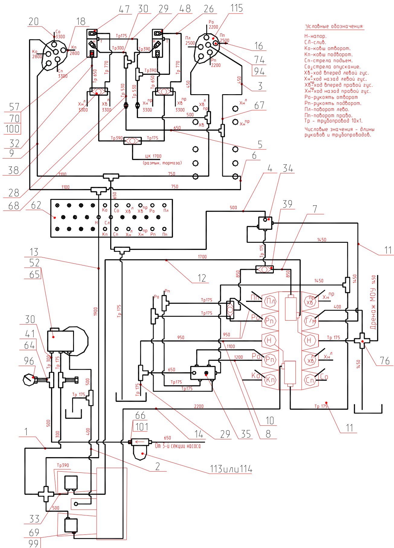
Рис. 35.1 Гидроуправление на поворотной платформе (монтажная схема) (с гидравликой ПСМ) Fig. 35.1 Hydraulic control on slewing turntable (assembly diagram) (PCM hydraulics)
