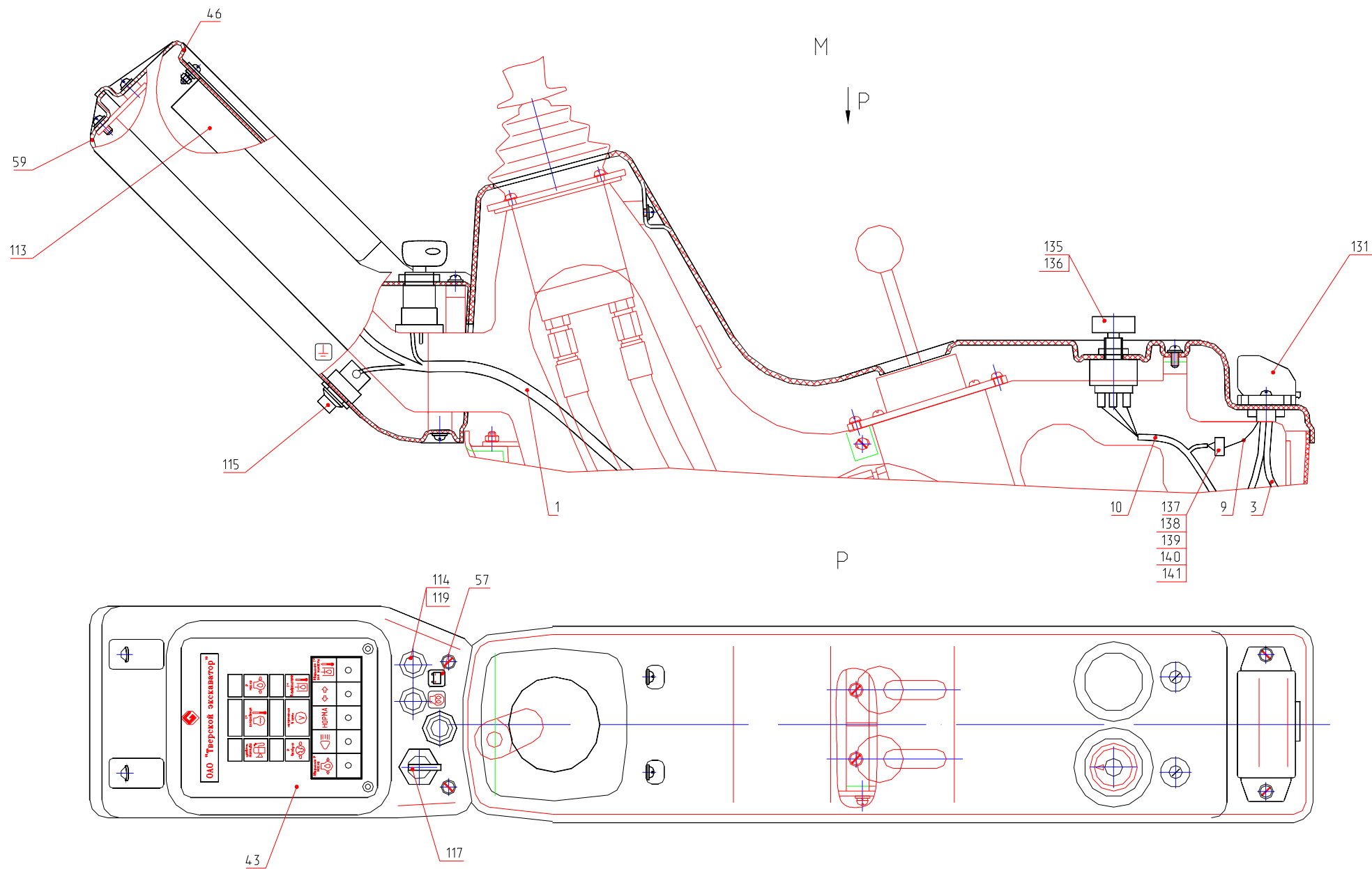
Рис. 62.4 Электрооборудование Fig. 62.4 Electric Equipment
