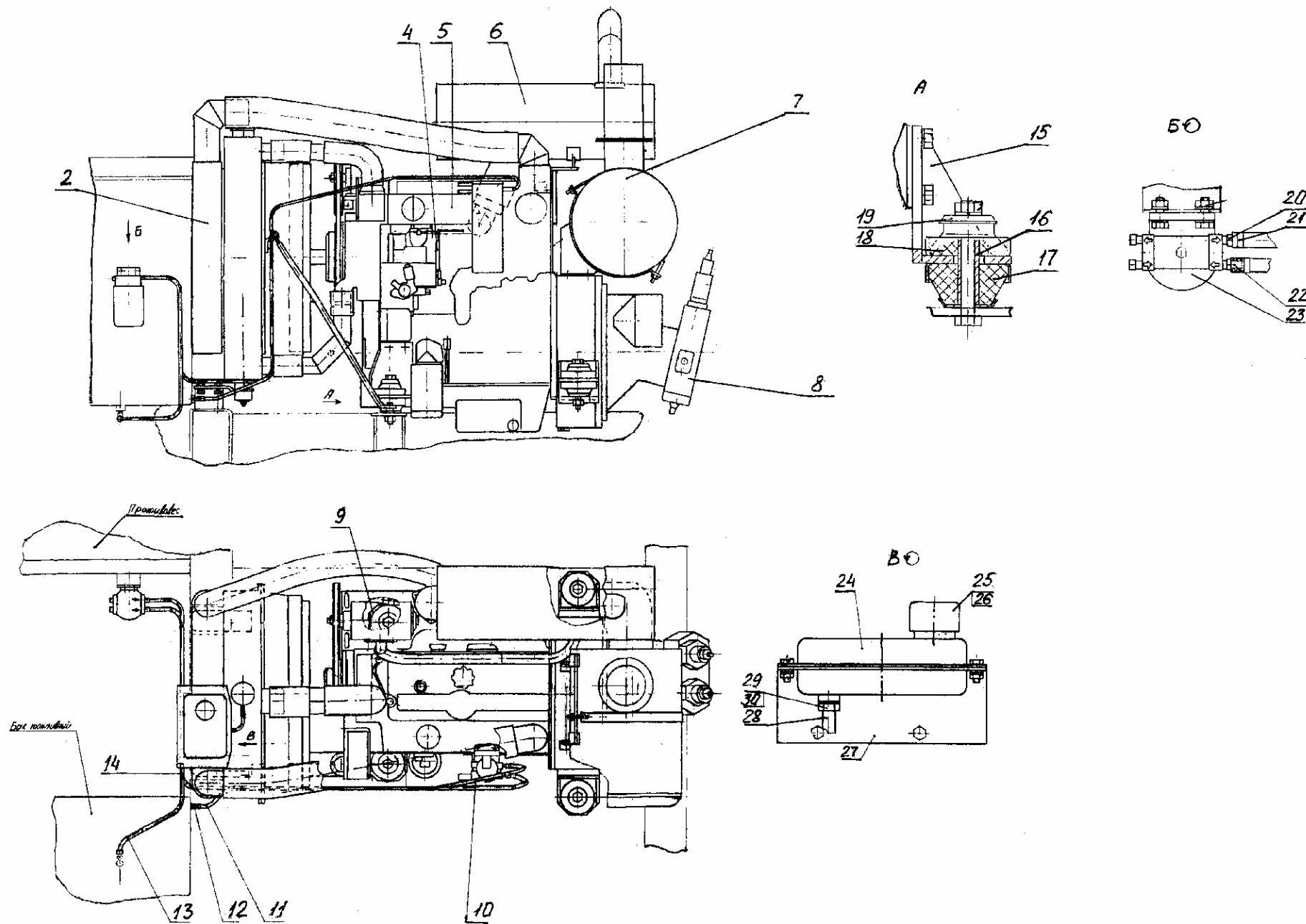
Рис. 8 Установка силовая
