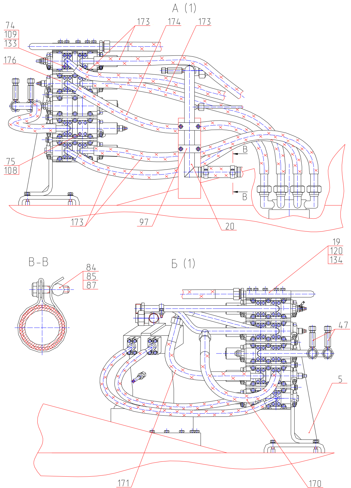
Рис. 28.2 Трубопроводы на поворотной платформе Fig. 28.2 Pipings on Slewing Turntable
