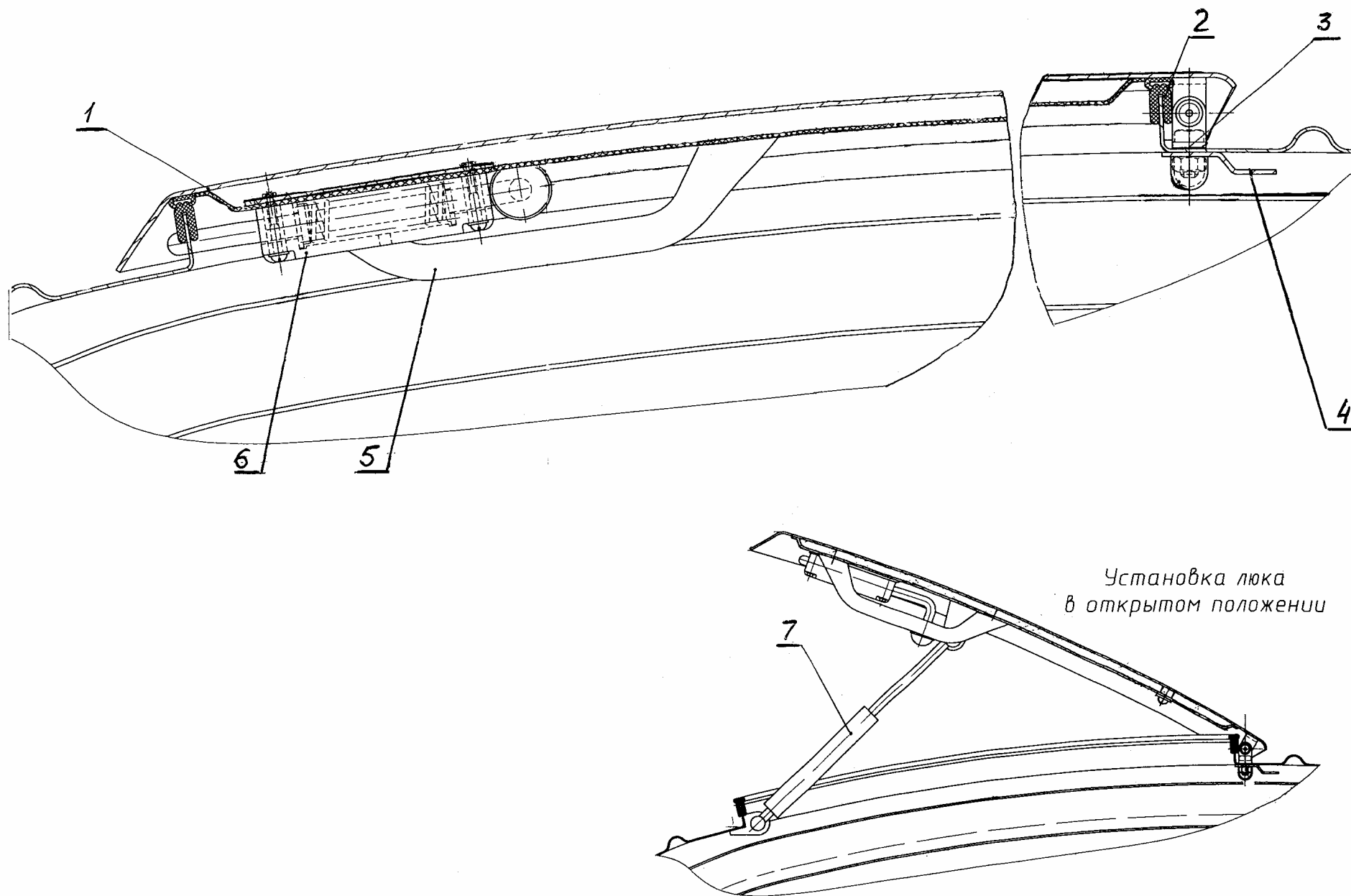
Рис. 15 Установка люка Fig. 15 Hatch Installation
