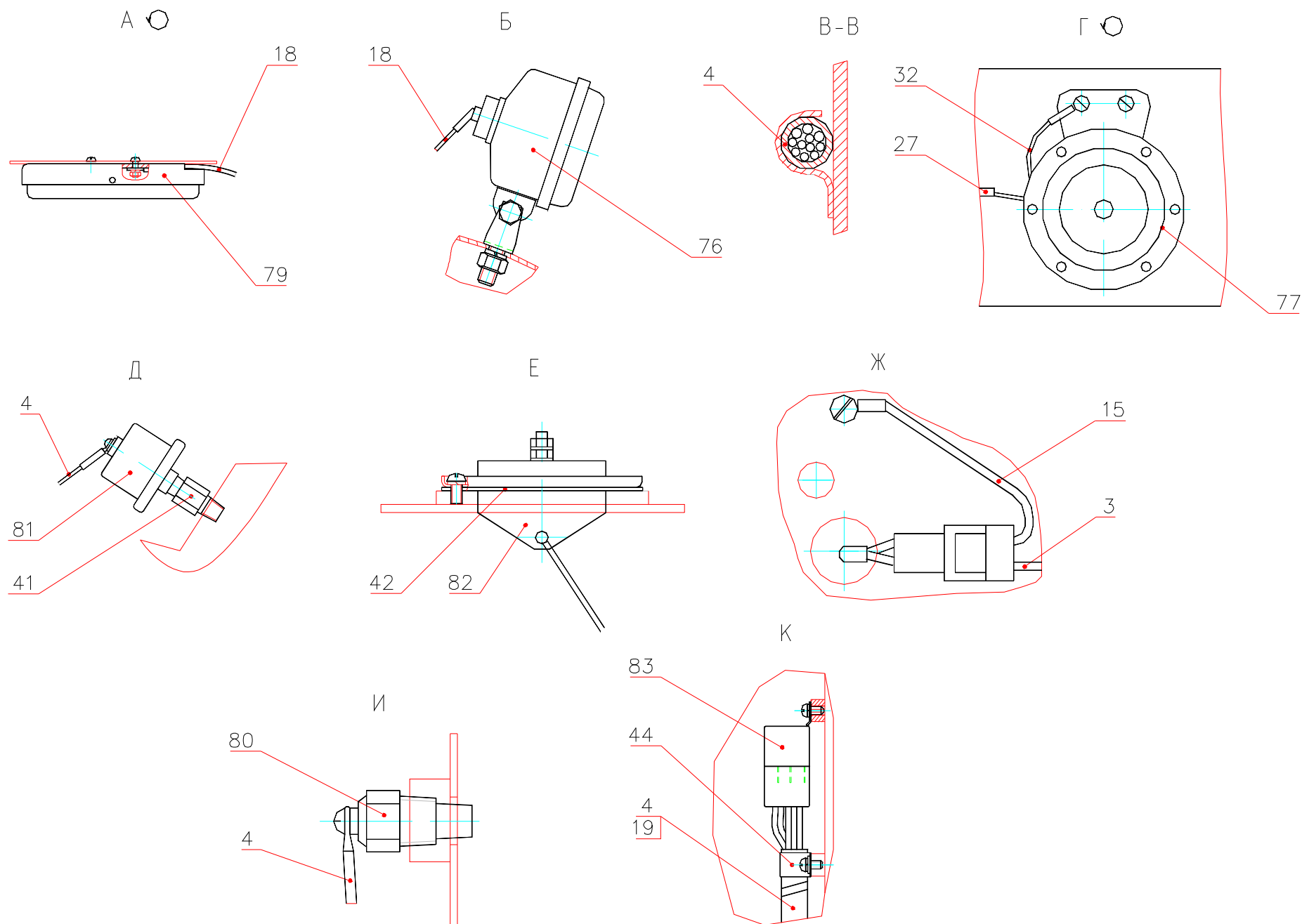
Рис. 61.3 Электрооборудование
