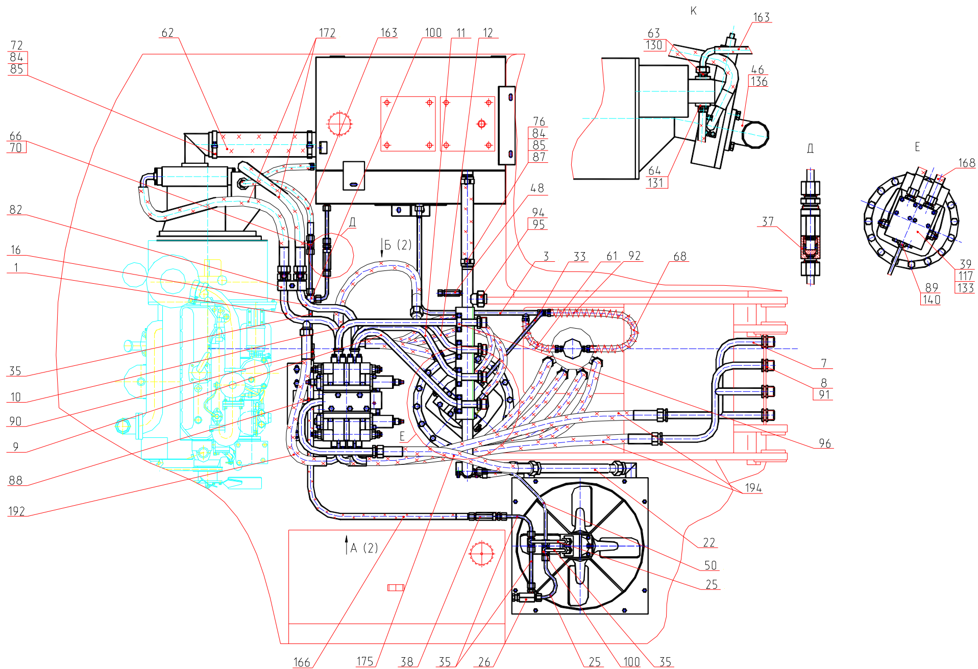
Рис. 28.1 Трубопроводы на поворотной платформе Fig. 28.1 Pippings on Slewing Turntable
