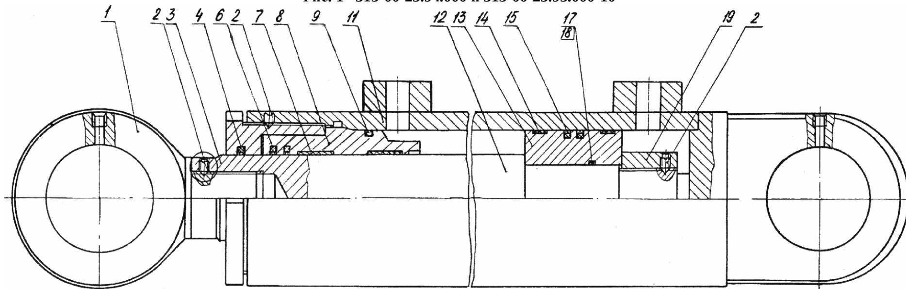
Рис. 2 313-00-23.94.000-11 и 313-00-23.95.000-11
