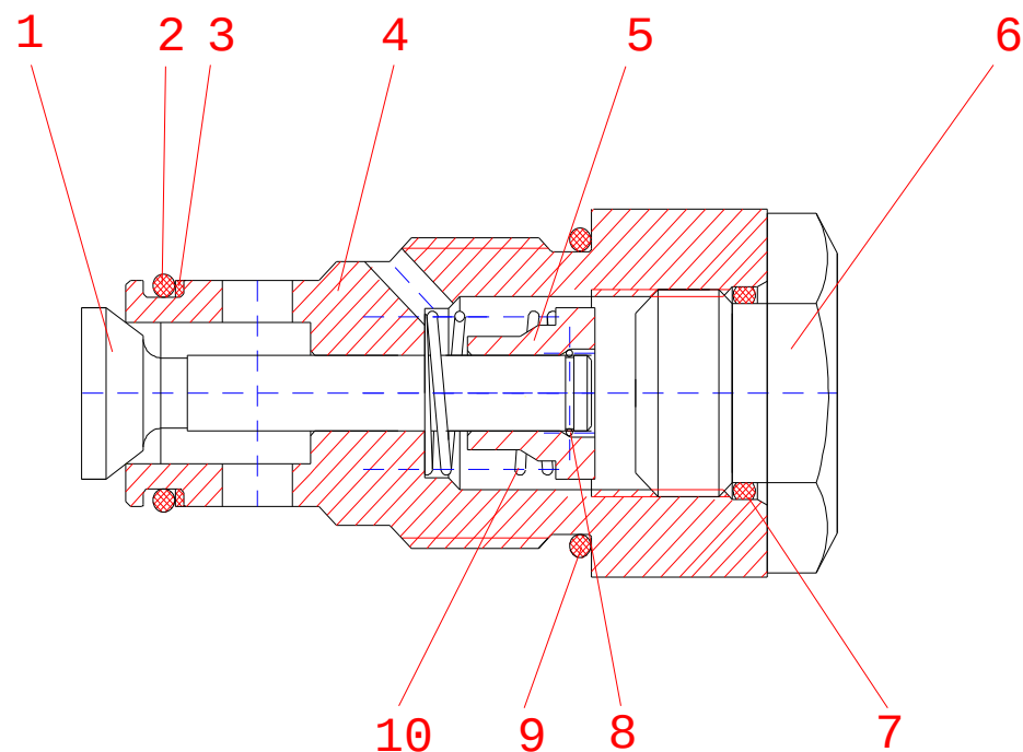
Рис. 34 Клапан подпиточный Fig. 34 Filling Valve
