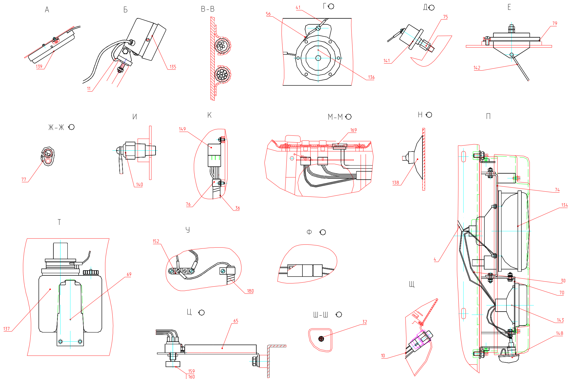
Рис. 47.3 Электрооборудование
