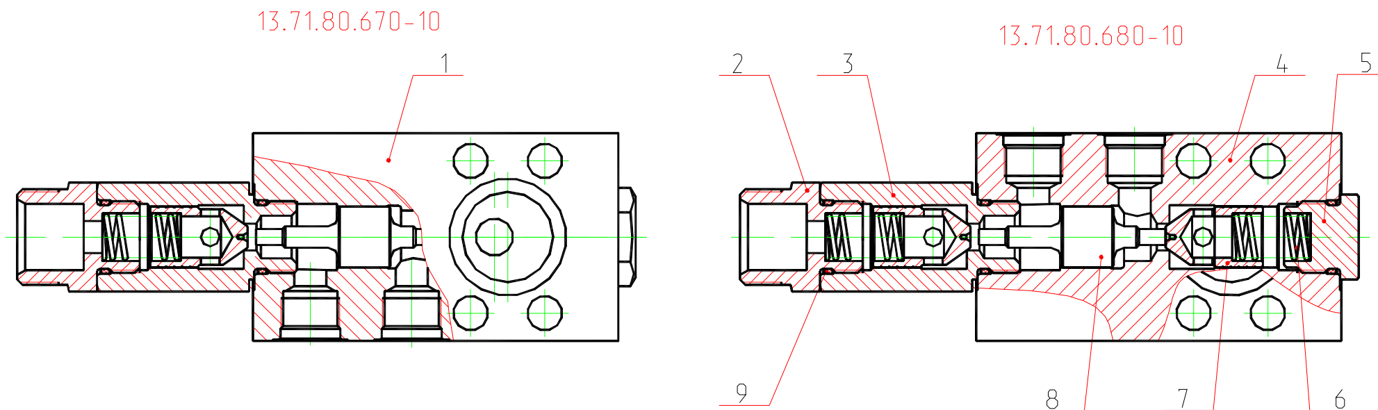
Рис. 60 Гидрозамок двухсторонний Fig. 60 Double-Sided Hydraulic Lock
