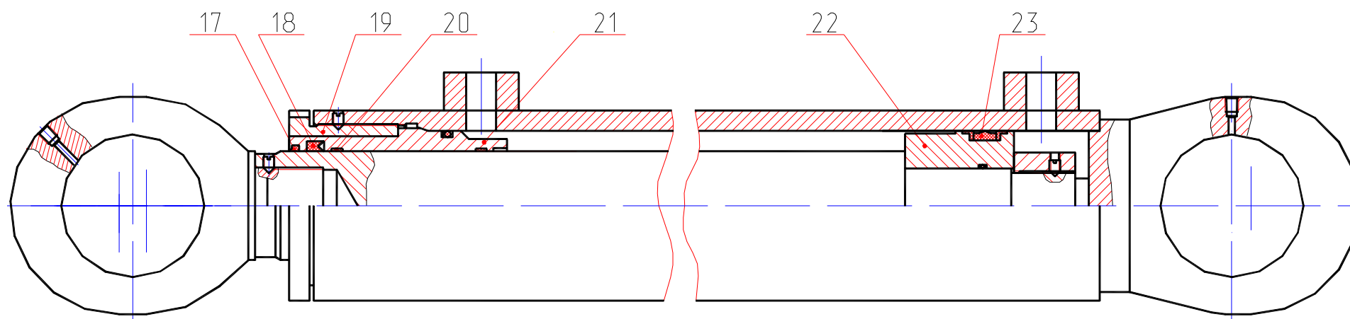
Рис. 51 Гидроцилиндр Fig. 51 Hydraulic Cylinder
