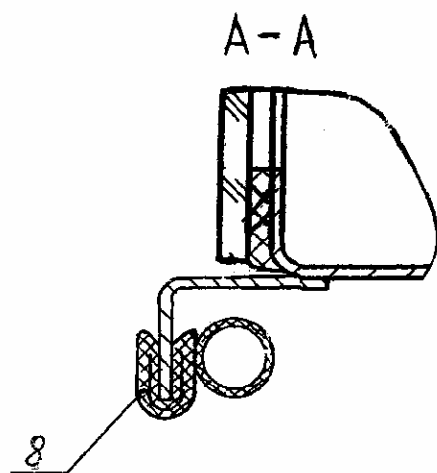
Рис. 15 Рамка верхняя Fig. 15 Upper Frame
