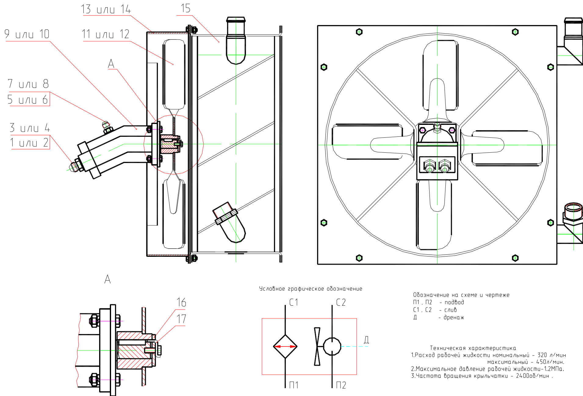
Рис. 44 Установка маслоохладительная Fig. 44 Oil Cooler Installation
