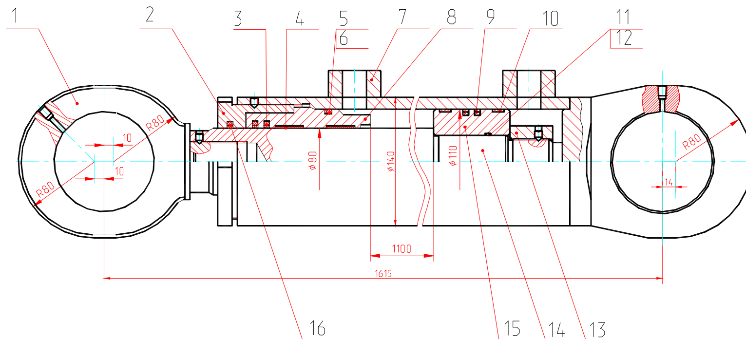
Рис. 2 100-80-11.02.000-11 Остальное см. рис. 1
