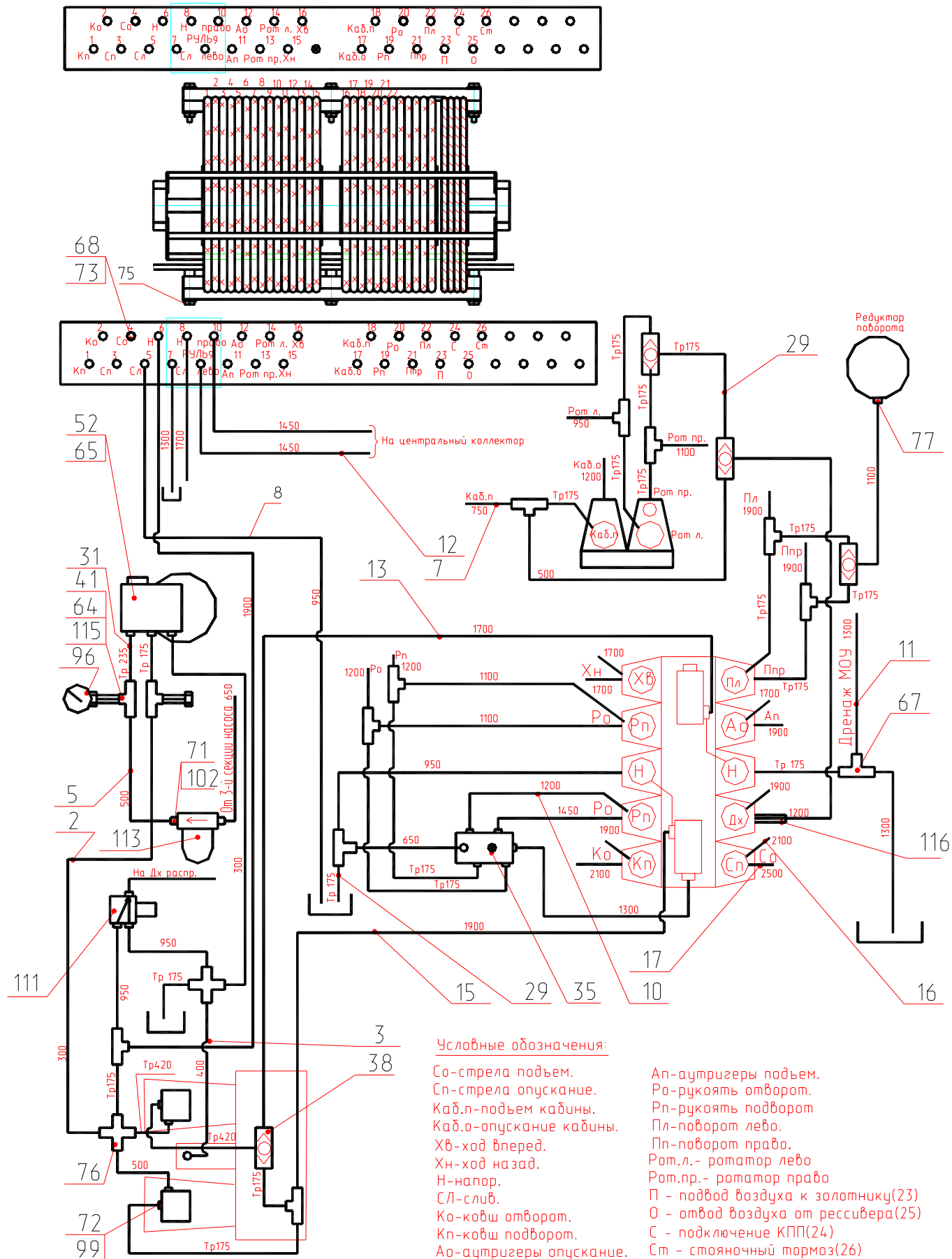
Рис. 34.2 Гидроуправление на поворотной платформе (монтажная схема) Fig. 34.2 Hydraulic control on slewing turntable (assembly diagram)
