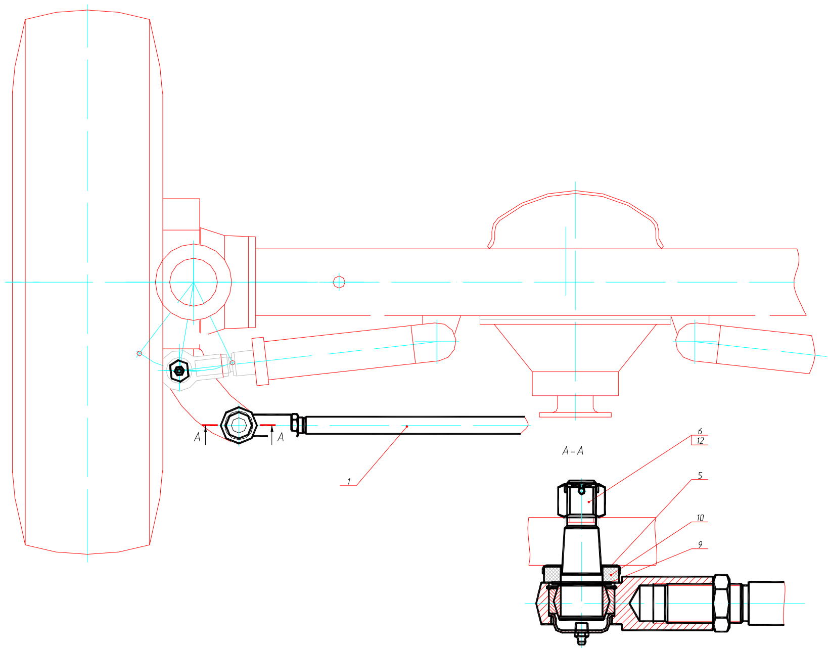
Рис. 69 Управление поворотом колес Fig. 69 Steering Gear
