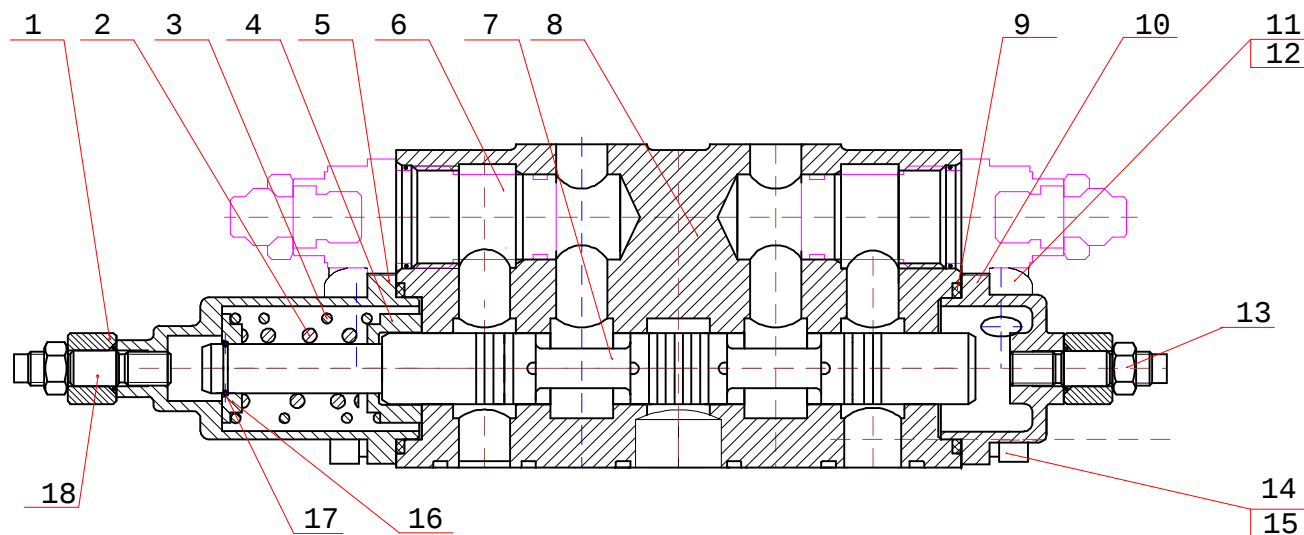
Рис. 32 Секция рабочая Fig. 32 Working Section
