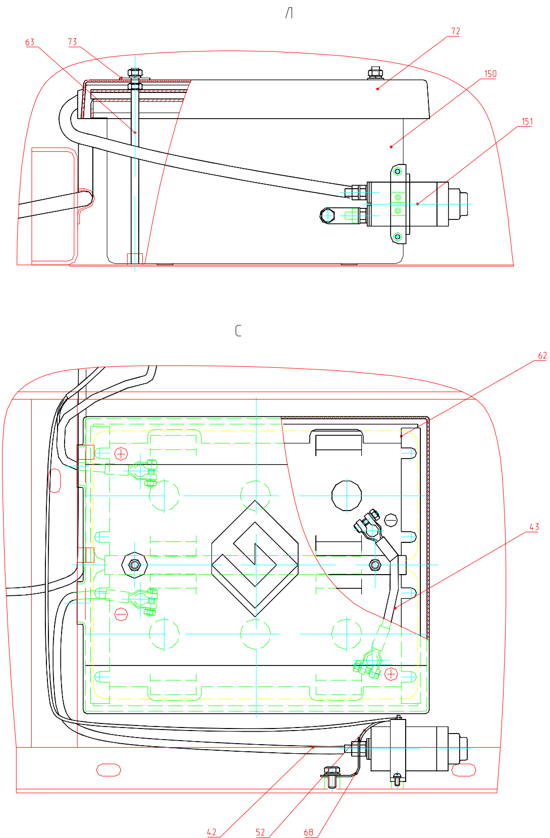
Рис. 47.4 Электрооборудование Fig. 47.4 Electric Equipment
