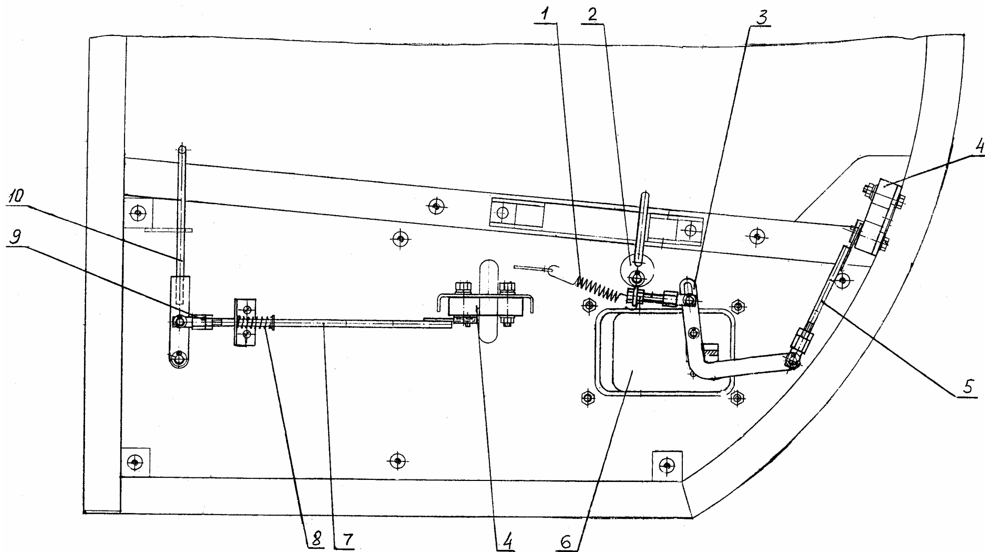
Рис. 13 Установка замков Fig. 13 Lock Installation
