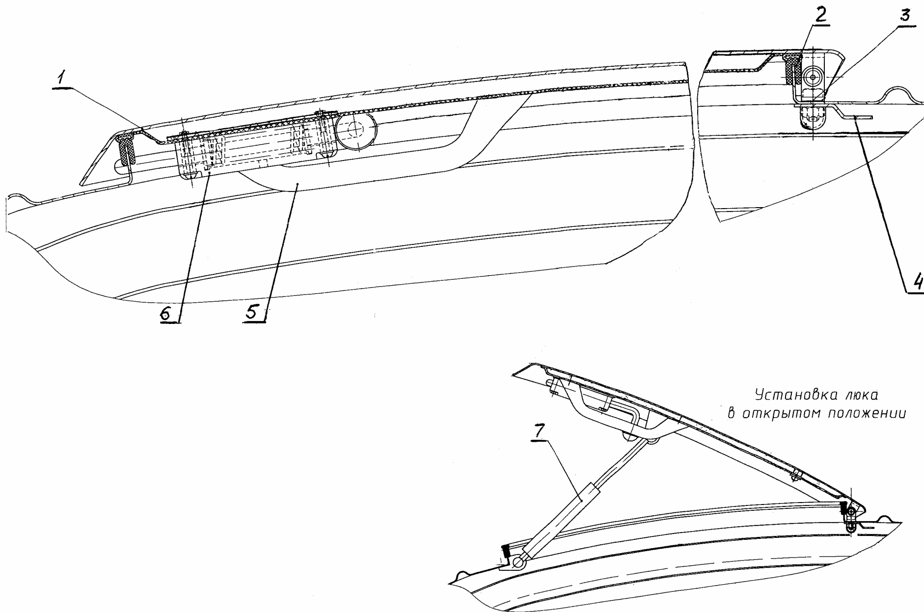
Рис. 11 Установка люка Fig. 11 Hatch Installation
