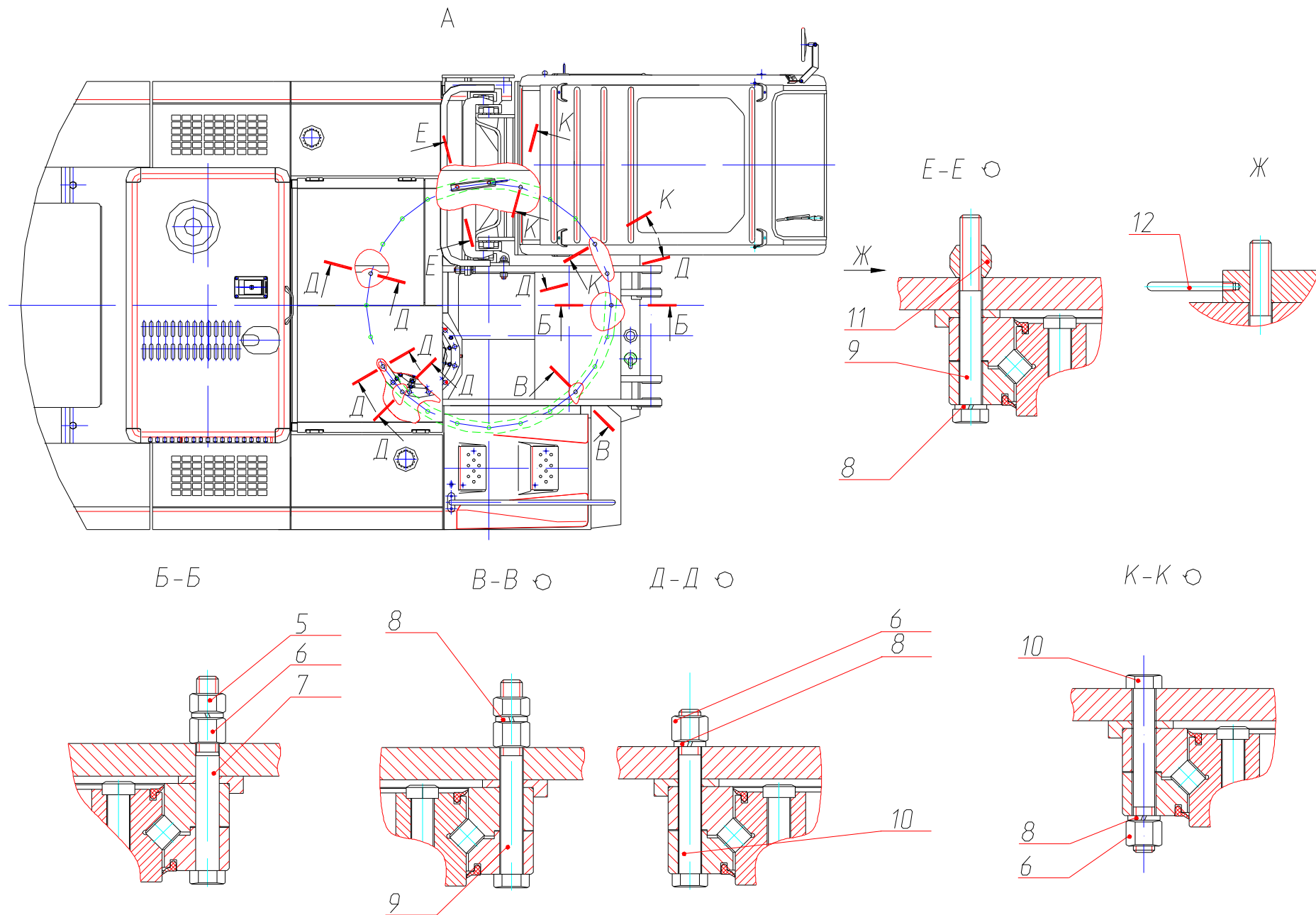
Рис. 1.2 Экскаватор пневмоколенный гидравлический с подъемной кабиной Fig. 1.2 Pneumatic-Tyred Hydraulic Excavator with Lifting Cab
