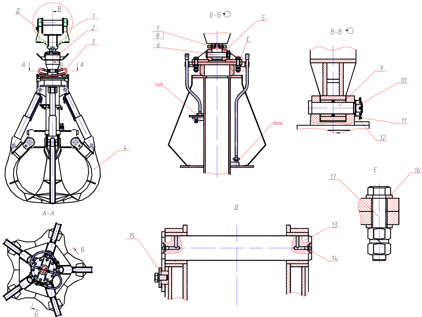
Рис. 53 Грейфер ГП-554 с ротатором РУ-80 Fig. 53 Grab with Rotator PY-80
