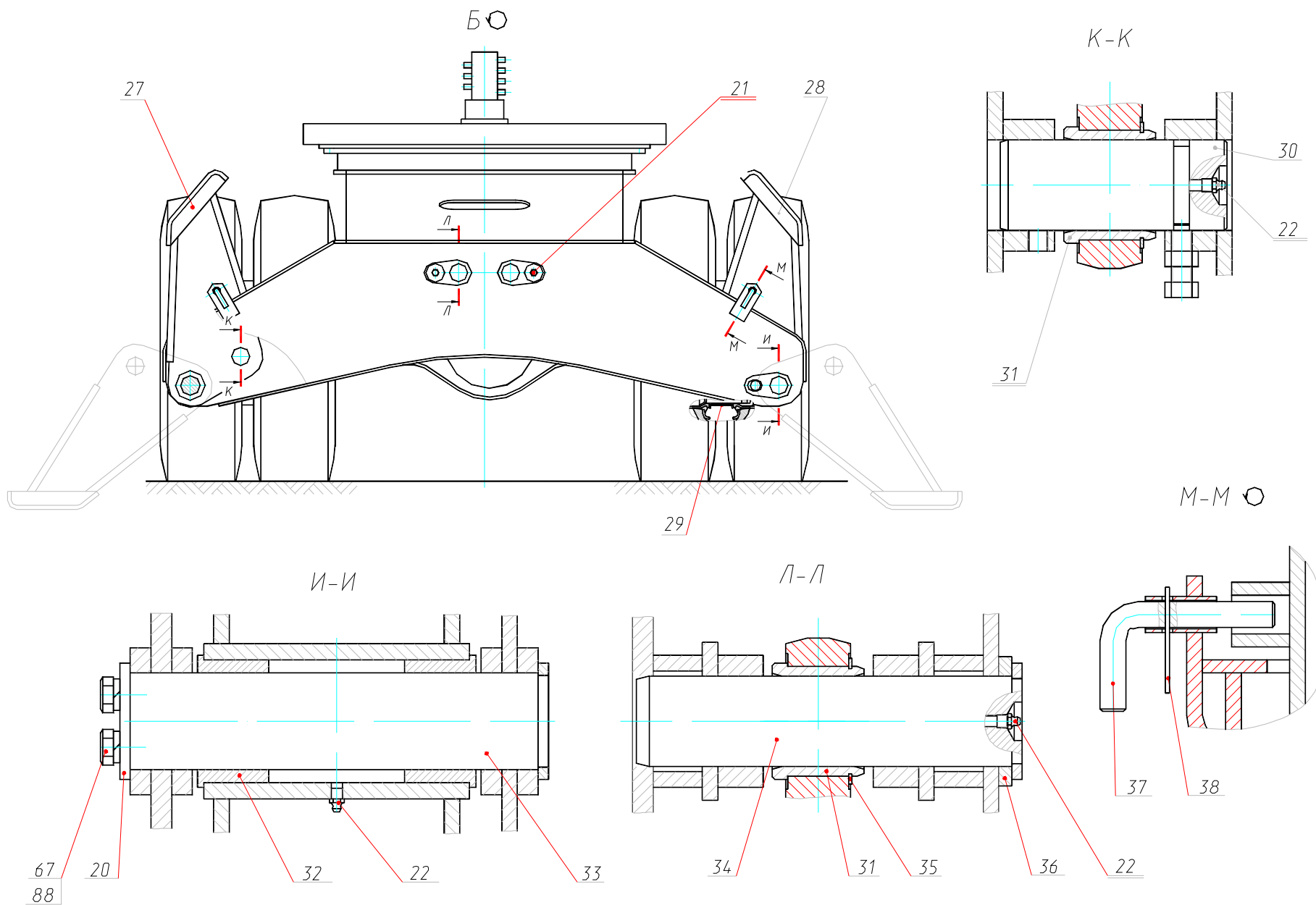
Рис. 56.3 Ход пневмоколесный Fig. 56.3 Pneumatic-Tyred Running Gear
