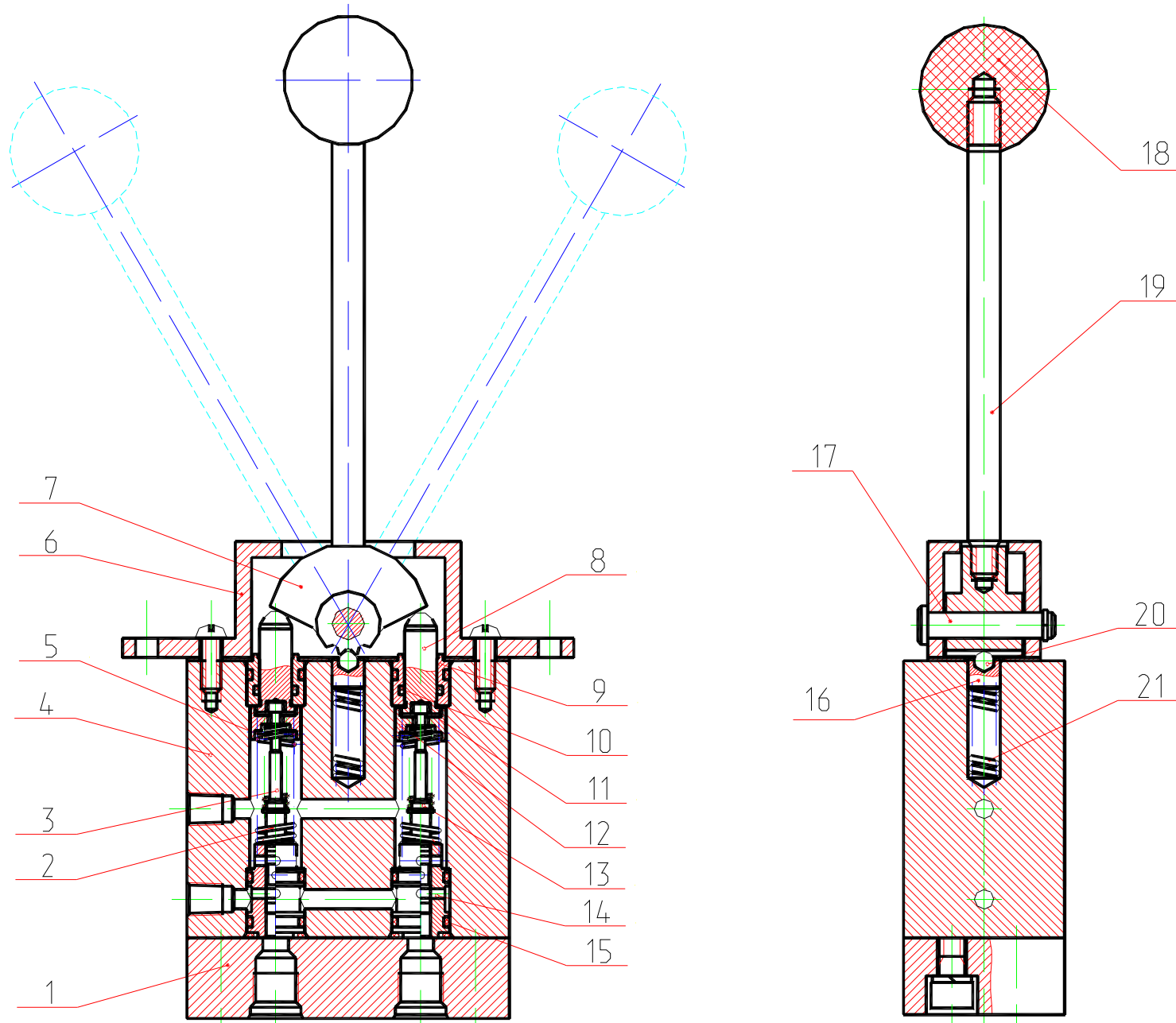
Рис. 39 Блок управления Fig. 39 Control Unit
