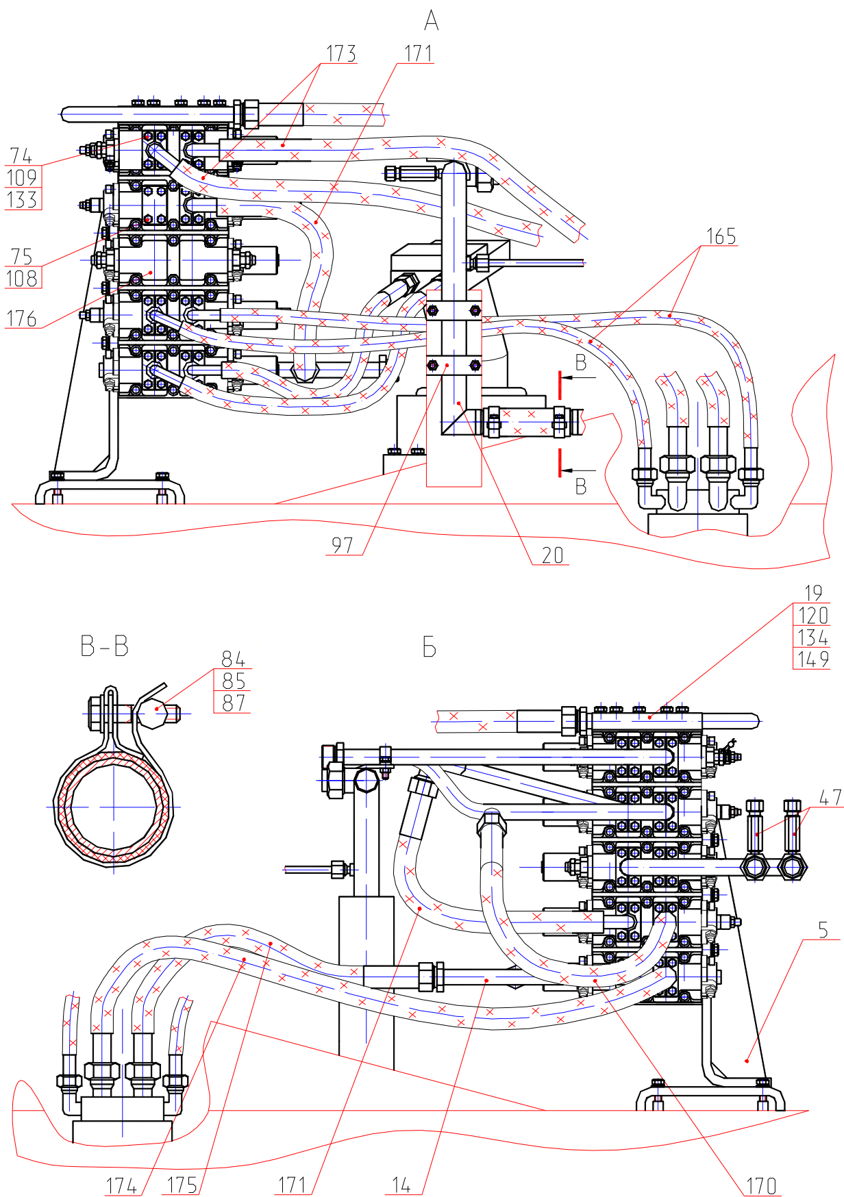
Рис. 21.26 Трубопроводы на поворотной платформе Fig. 21.26 Pipings on Slewing Turntable
