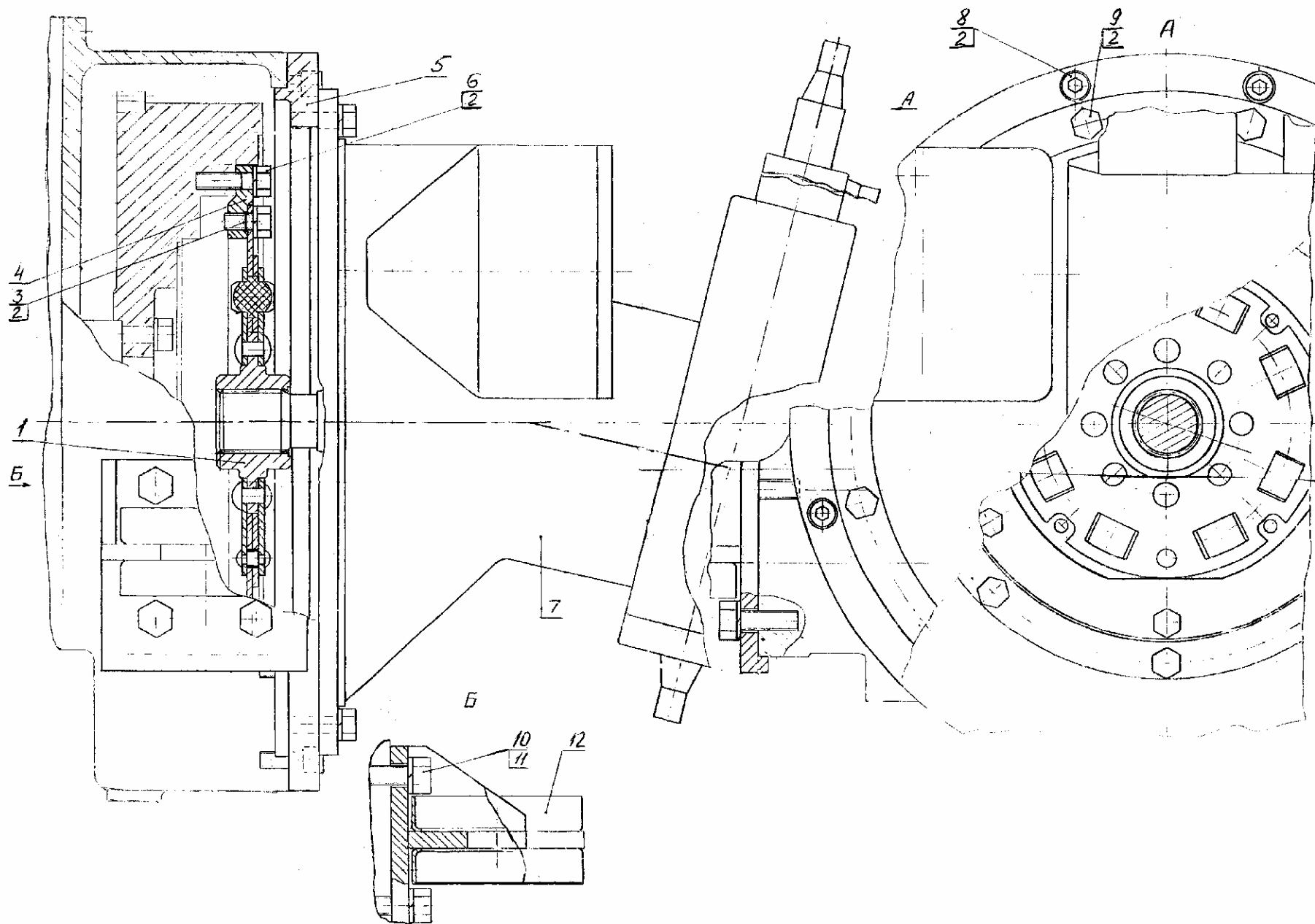
Рис. 76 Установка насоса Fig. 76 Pump Installation 182
