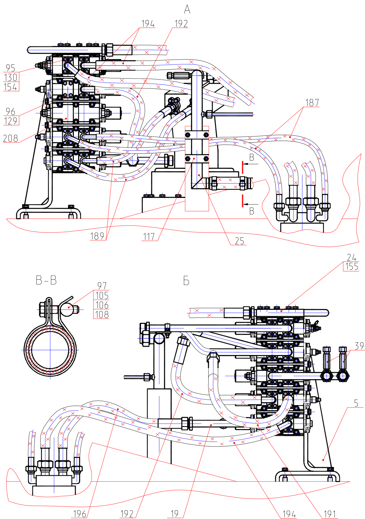
Рис. 21.2a Трубопроводы на поворотной платформе Fig. 21.2a Pippings on Slewing Turntable
