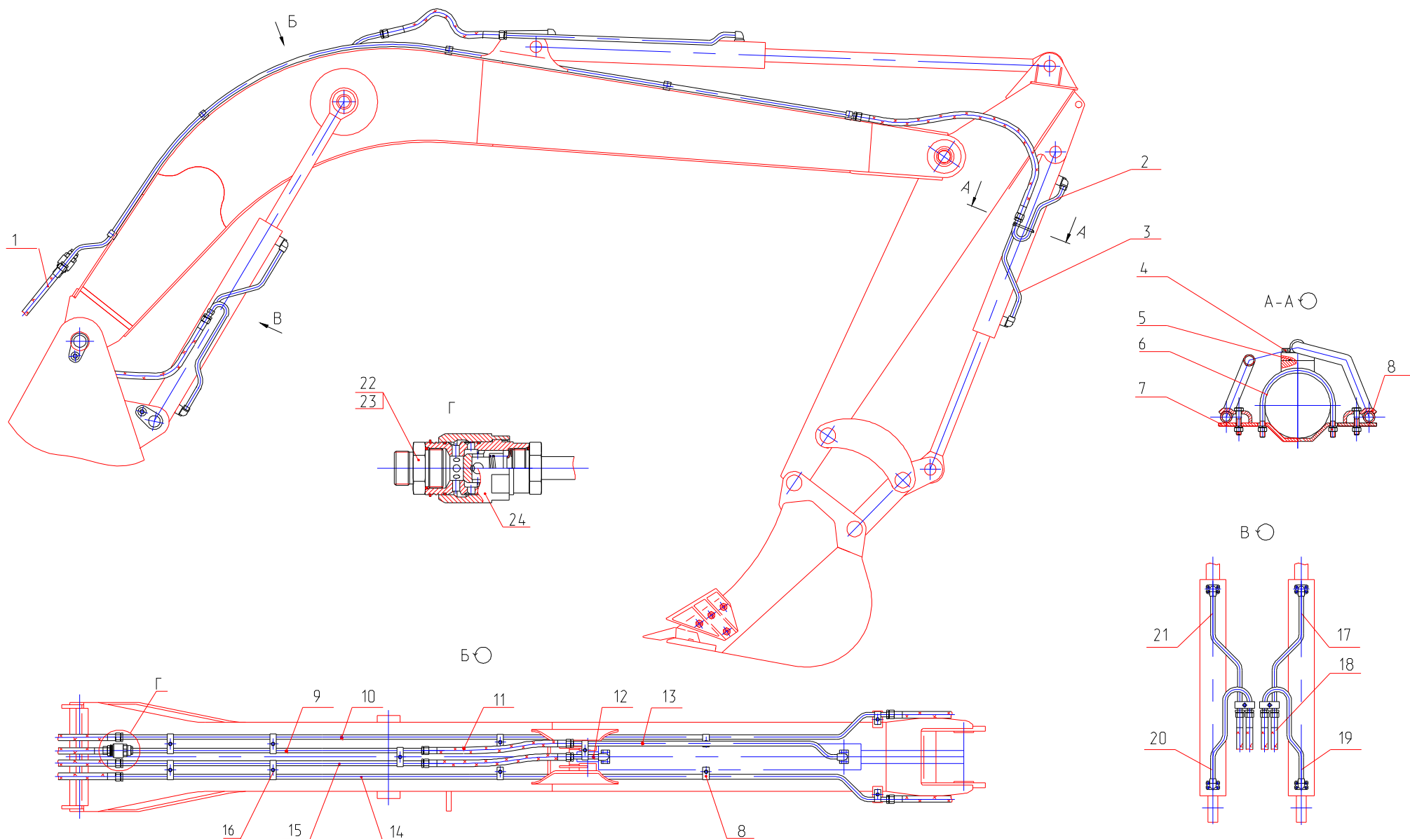
Рис. 42 Трубопроводы рабочего оборудования Fig. 42 Backhoe Equipment Pipings
