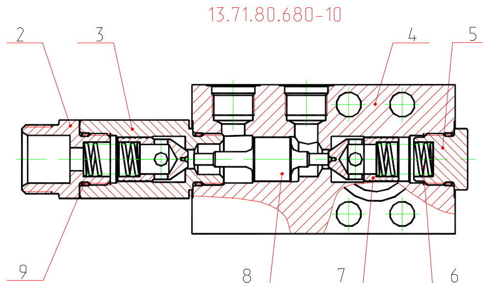
Рис. 51 Гидрозамок двухсторонний Fig. 51 Double-Sided Hydraulic Lock
