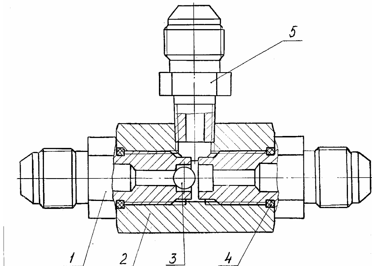
Рис. 32 Клапан «ИЛИ» Fig. 32 Valve «OR»
