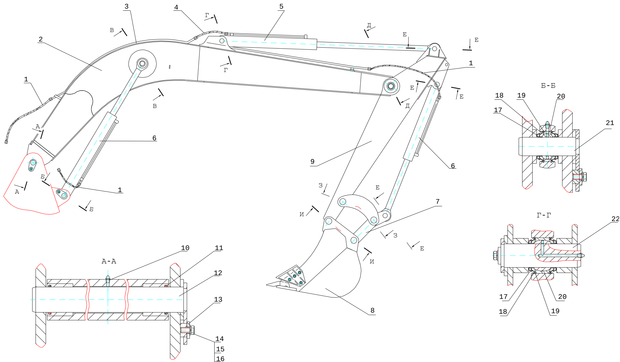
Рис. 41.1 Рабочее оборудование обратной лопаты Fig. 41.1 Backhoe Equipment
