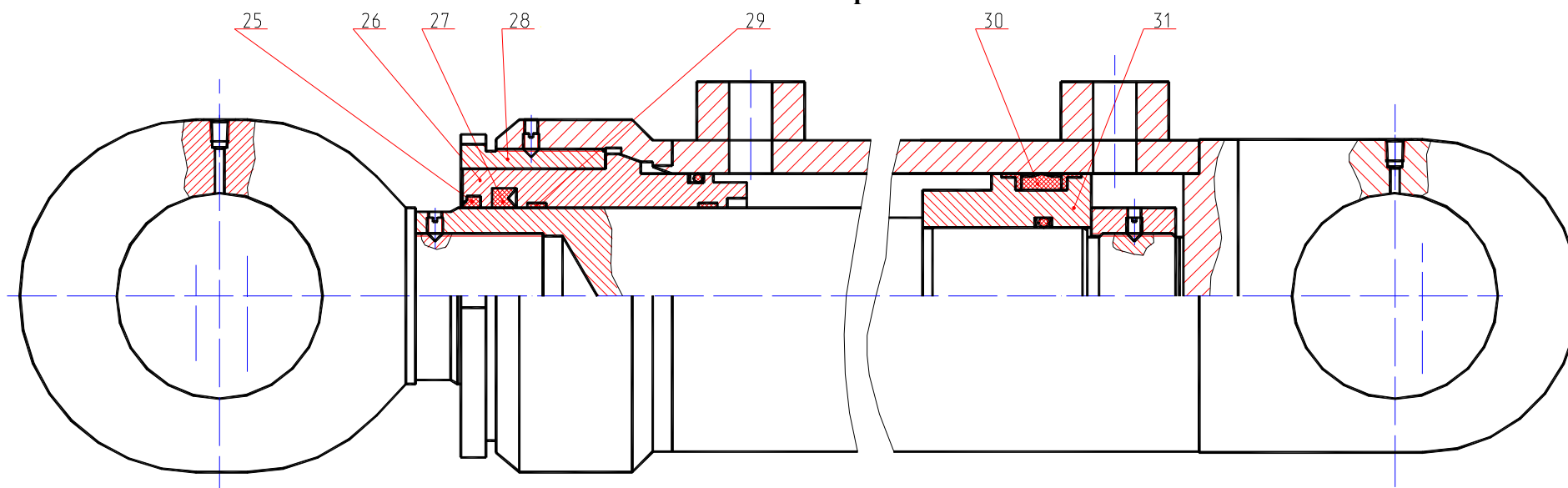
Рис. 43 Гидроцилиндр рукояти
