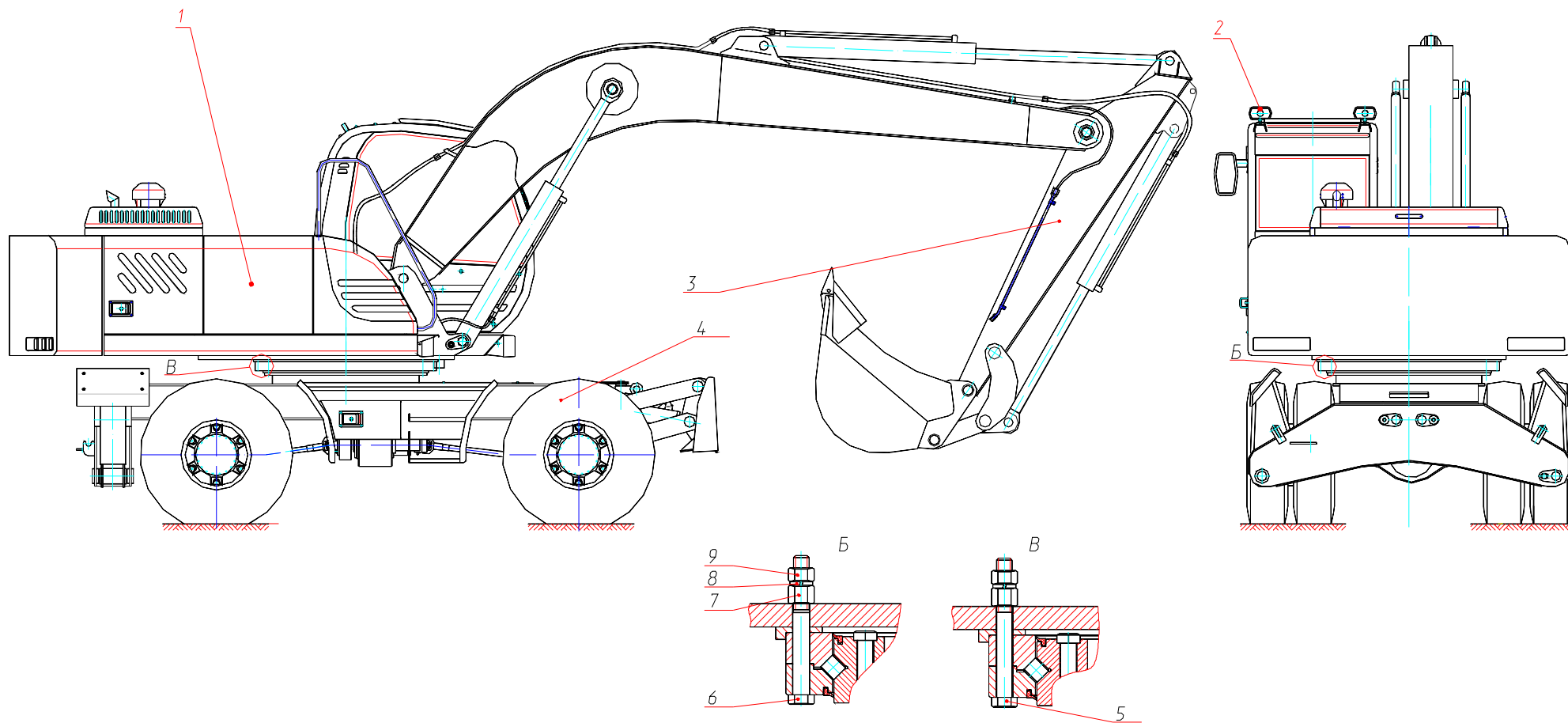
Рис. 1 Экскаватор пневмоколесный гидравлический Fig. 1 Single-Bucket Pneumatic-Tyred Hydraulic Excavator
