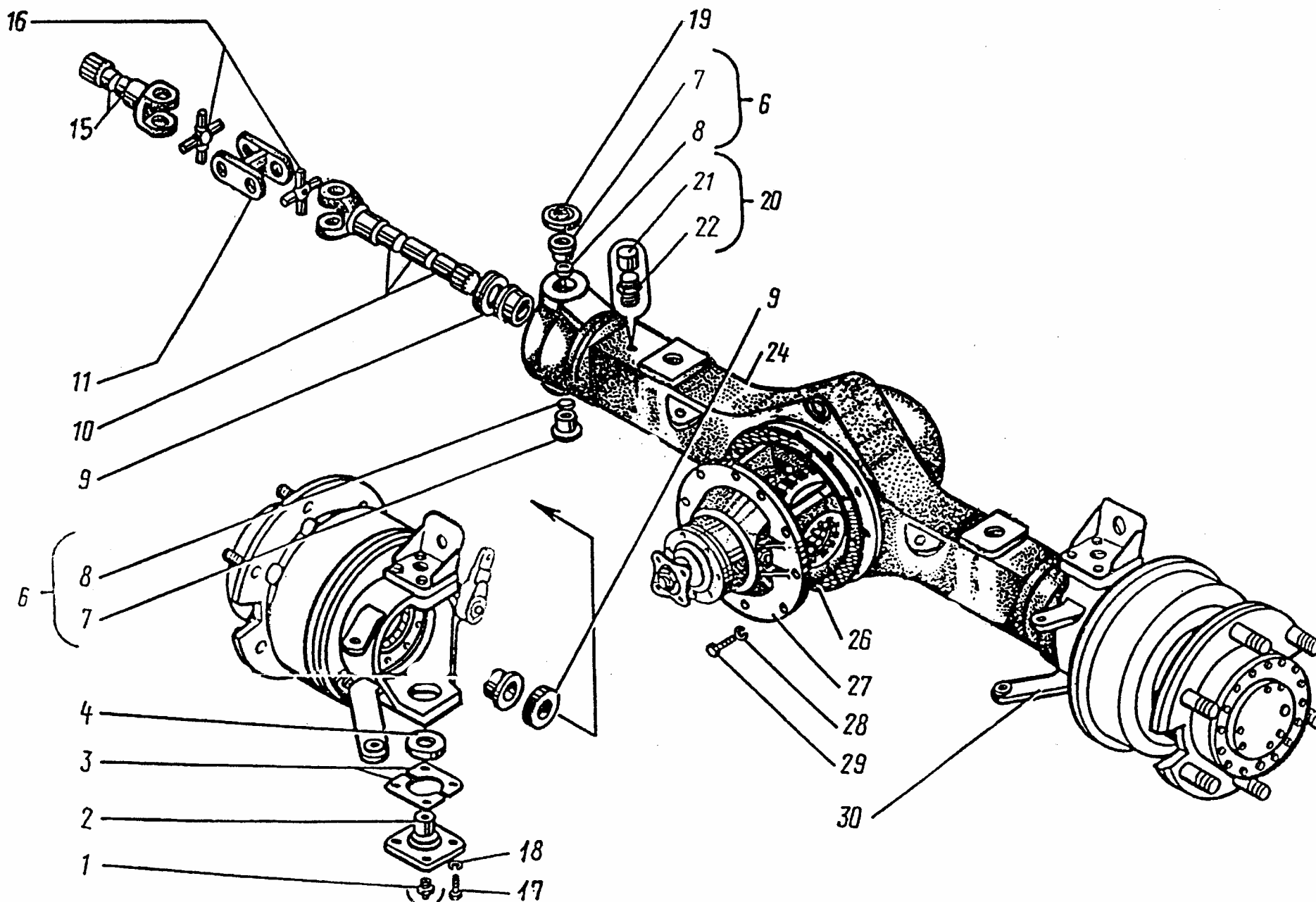
Рис. 62.1 Мост приводной управляемый Fig. 62.1 Driven Steer Axle
