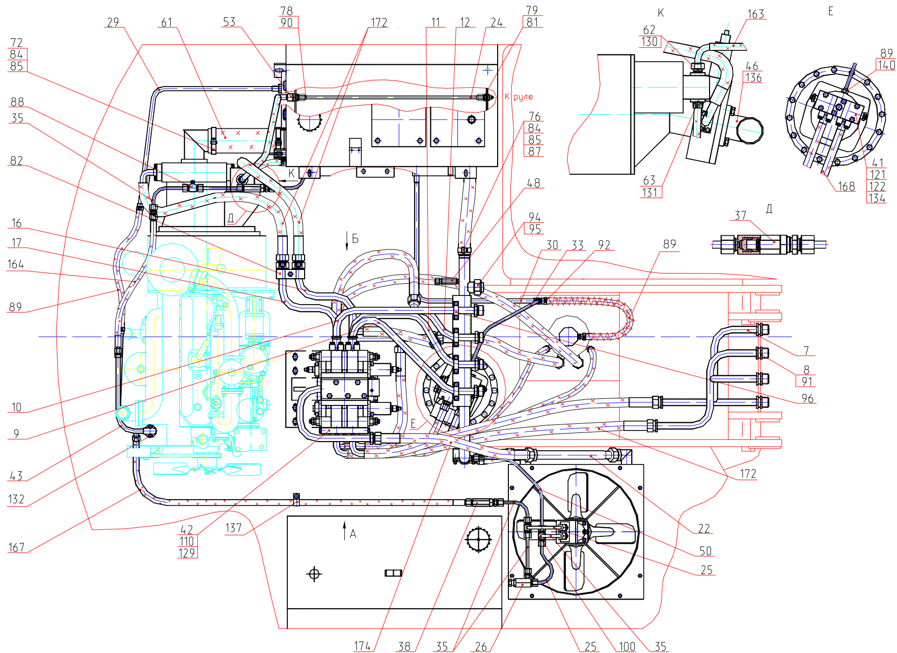
Рис. 21.16 Трубопроводы на поворотной платформе Fig. 21.16 Pipings on Slewing Turntable
