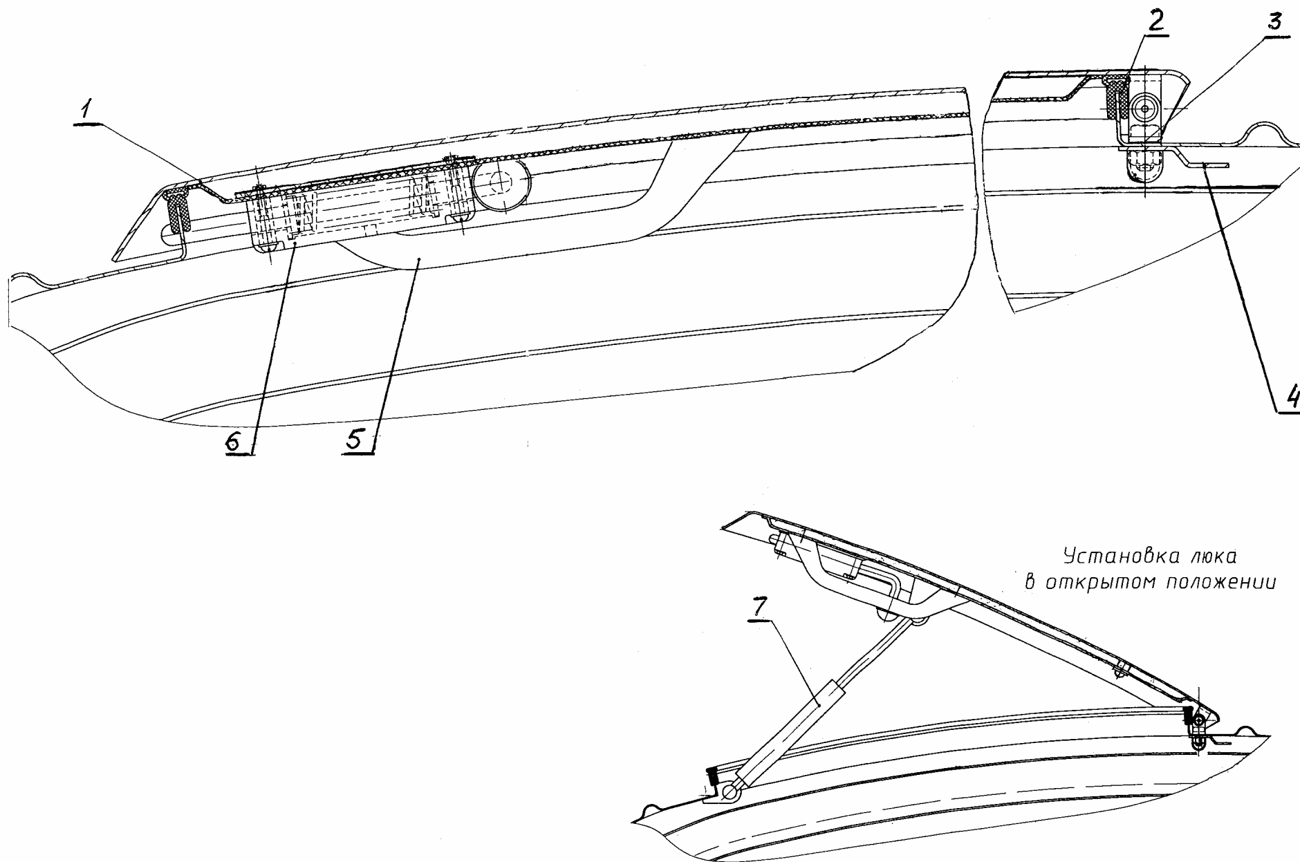
Рис. 6 Установка люка Fig. 6 Hatch Installation
