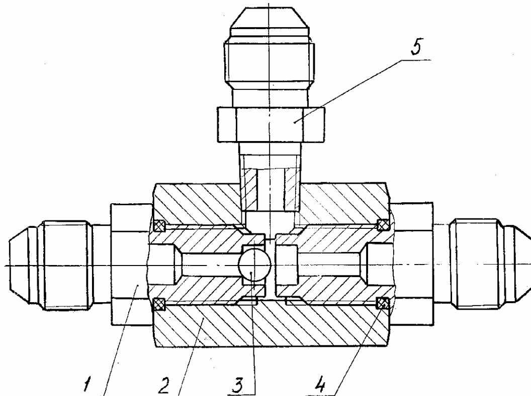
Рис. 22 Клапан «ИЛИ» Fig. 22 Valve «OR»
