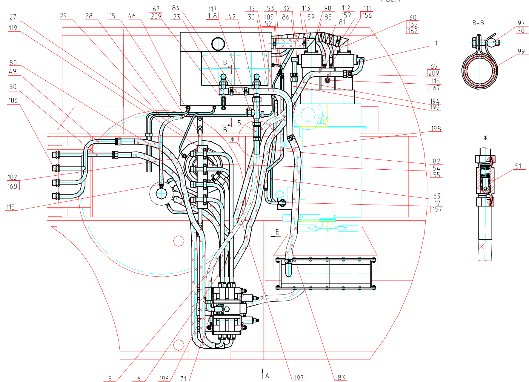
Рис. 8.1 Трубопроводы на поворотной платформе Fig. 8.1 Piping on Slewing Turntable 23
