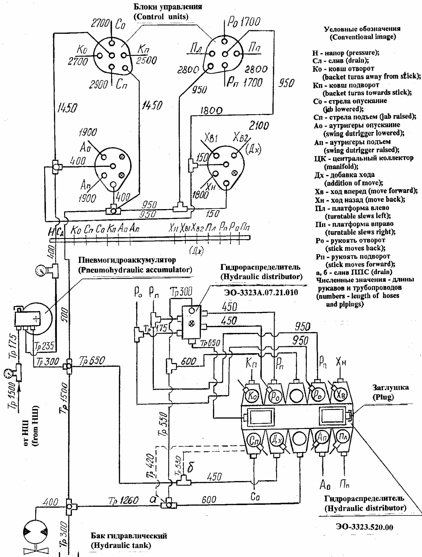
Рис. 18.3 Монтажная схема гидроуправления Fig. 18.3 Hydraulic Control Assembly Diagram
