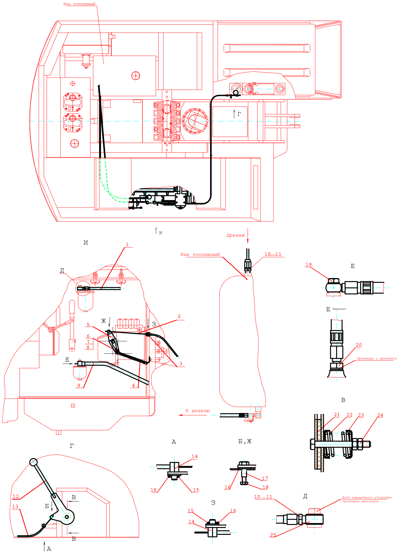
Рис. 39 Топливопроводы и управление подачей топлива Fig. 39 Fuel Piping and Fuel Supply Control System
