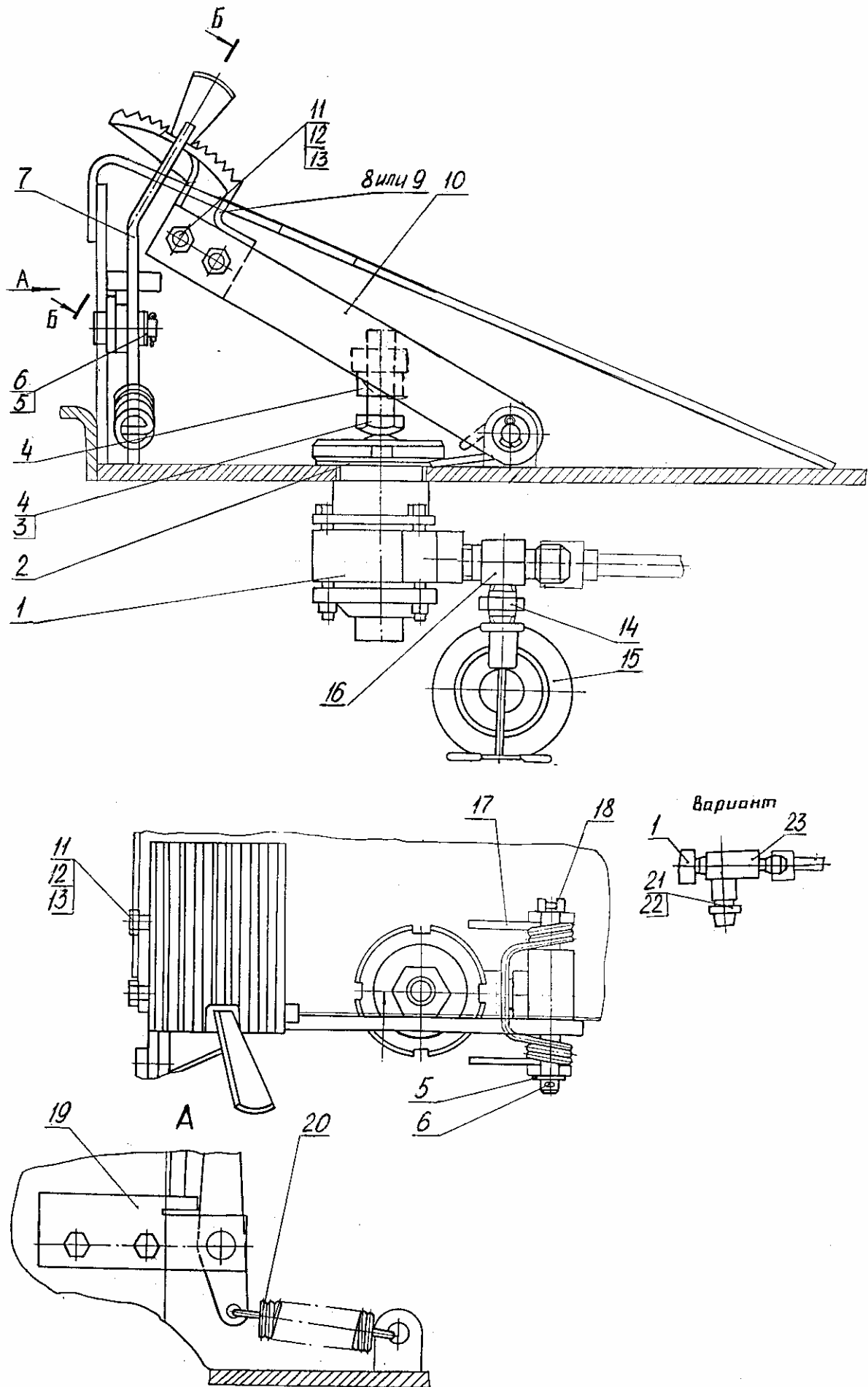
Рис. 14 Установка педали тормоза хода
