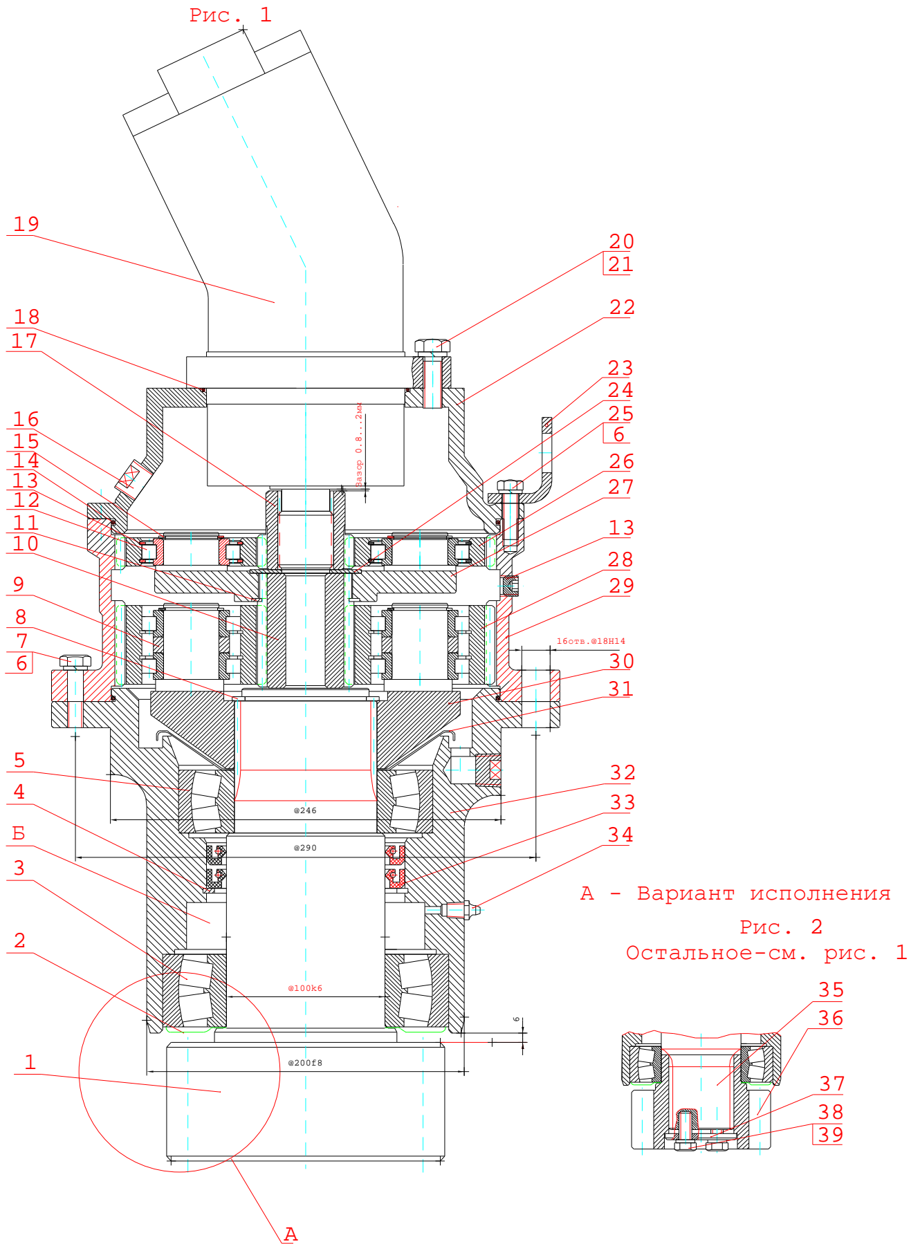
Рис. 5 Механизм поворота Fig. 5 Slewing Mechanism
